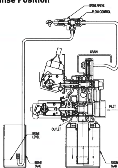
5 Rapid Rinse
